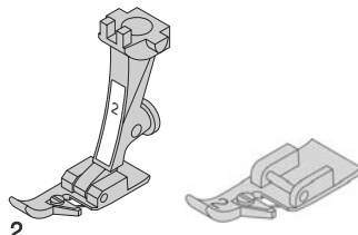
2 Оверлочная лапка/ Подошва оверлочной лапки * Оверлочные швы, подшивка с обметыванием среза, обметывание швов
