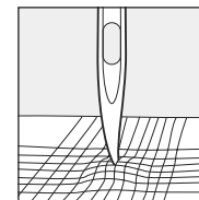
Острие с "крючком"
