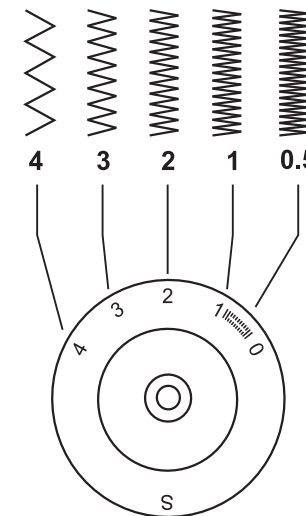
Регулятор длины стежка
