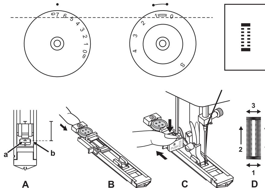
Регулятор ширины стежка
