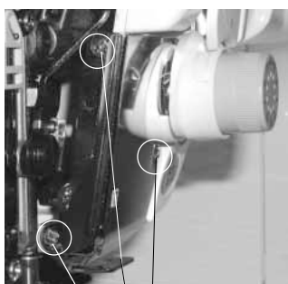
Setscrew (D)
