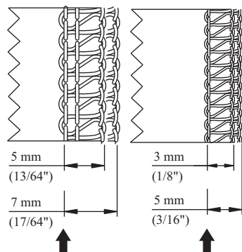
Левая игла
