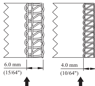
Левая игла
