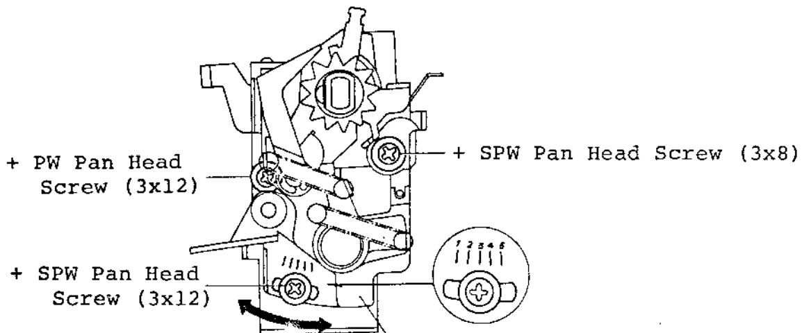
www.PromElectroAutomat.ru Fig. 66 Stop Lever Holder
