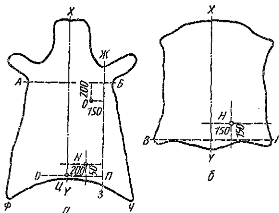
Рис. 111.4. Расположение точек H и O замера толщины и сбежистости на юфты из конских передин и полупереди (а), свиных шкур в виде целых кож и рыбок (б)
