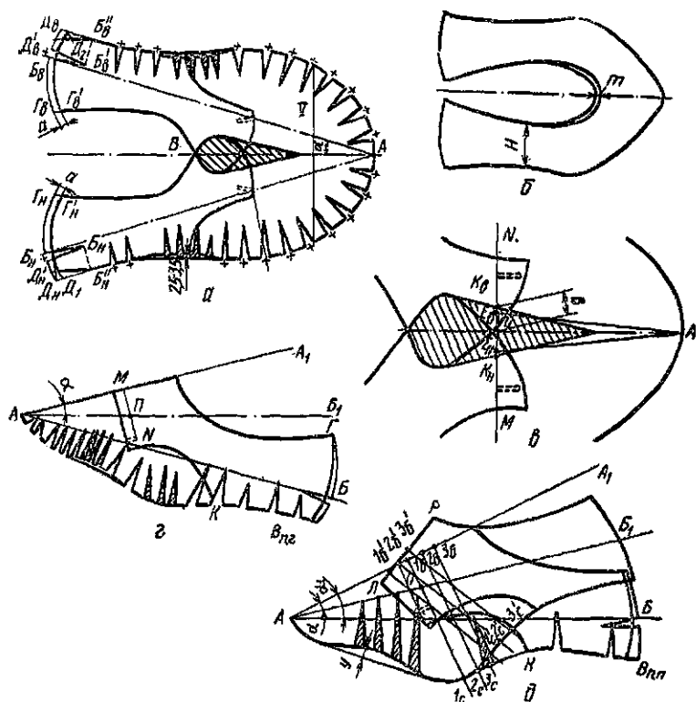
Рис. 11.31. Схема получения условной развертки полуплоских и плоских заготовок верха обуви со свободной затяжной кромкой
