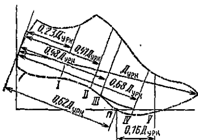
Рис. 11.28. Способ Ю. П. Зыбина нанесения базисных линий на копию колодки
