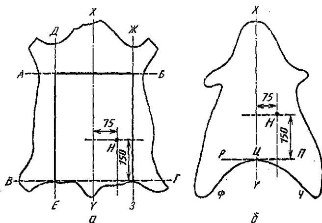
Рис. 111.5. Расположение точки H замера толщины целых кож и полукож хромового дубления, лаковых, замши, подкладочных (а), передин и полупереди хромового дубления для верха обуви (б): РП — касательная, проведенная через точку Ц к линии отделения хаза ФЦЧ
