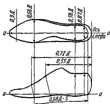
Рис. 11.19. Схема расположения наколов для проверки обхватов колодки
