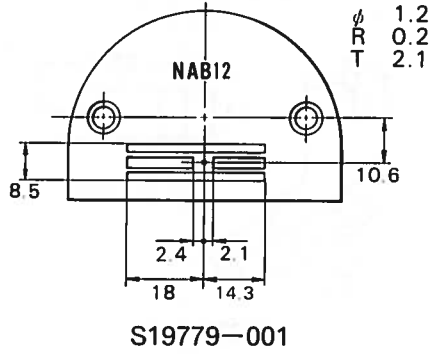
針 板 Needle Plate
