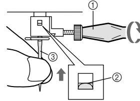
① Отвертка ② Ограничитель иглы ③ Игла
