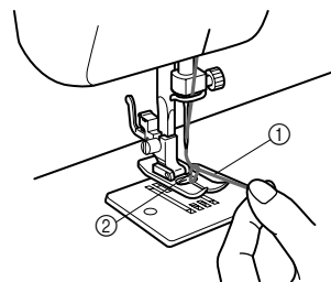
① Верхняя нить ② Петля нижней нити
