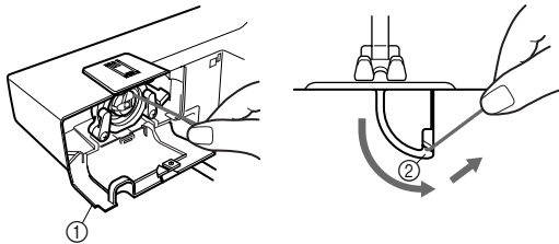
① Крышка челночного устройства ② Прорез
