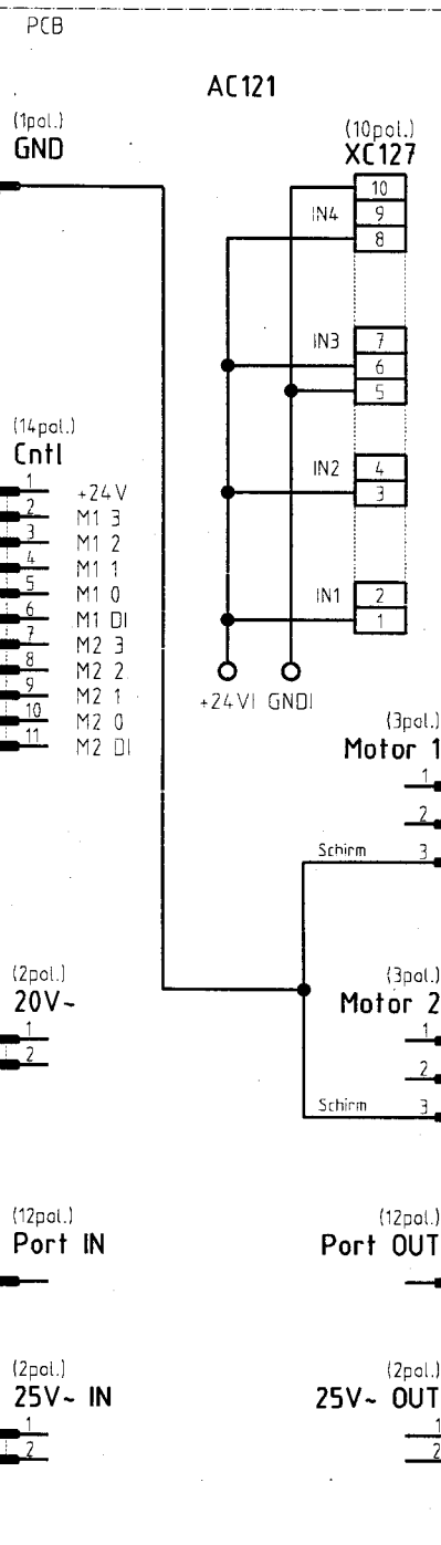
Leiterplatte k 9850 001051
