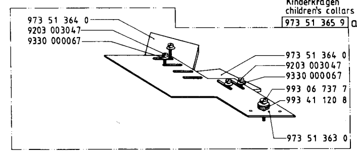
Fest-Anschlag rigid stop
