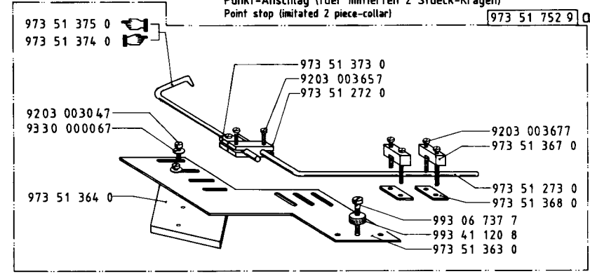
Punkt-Anschlag (fuer imitierten 2 Stueck-Kragen) Point stop (imitated 2 piece-collar)
