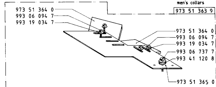
Fest-Anschlag rigid stop
